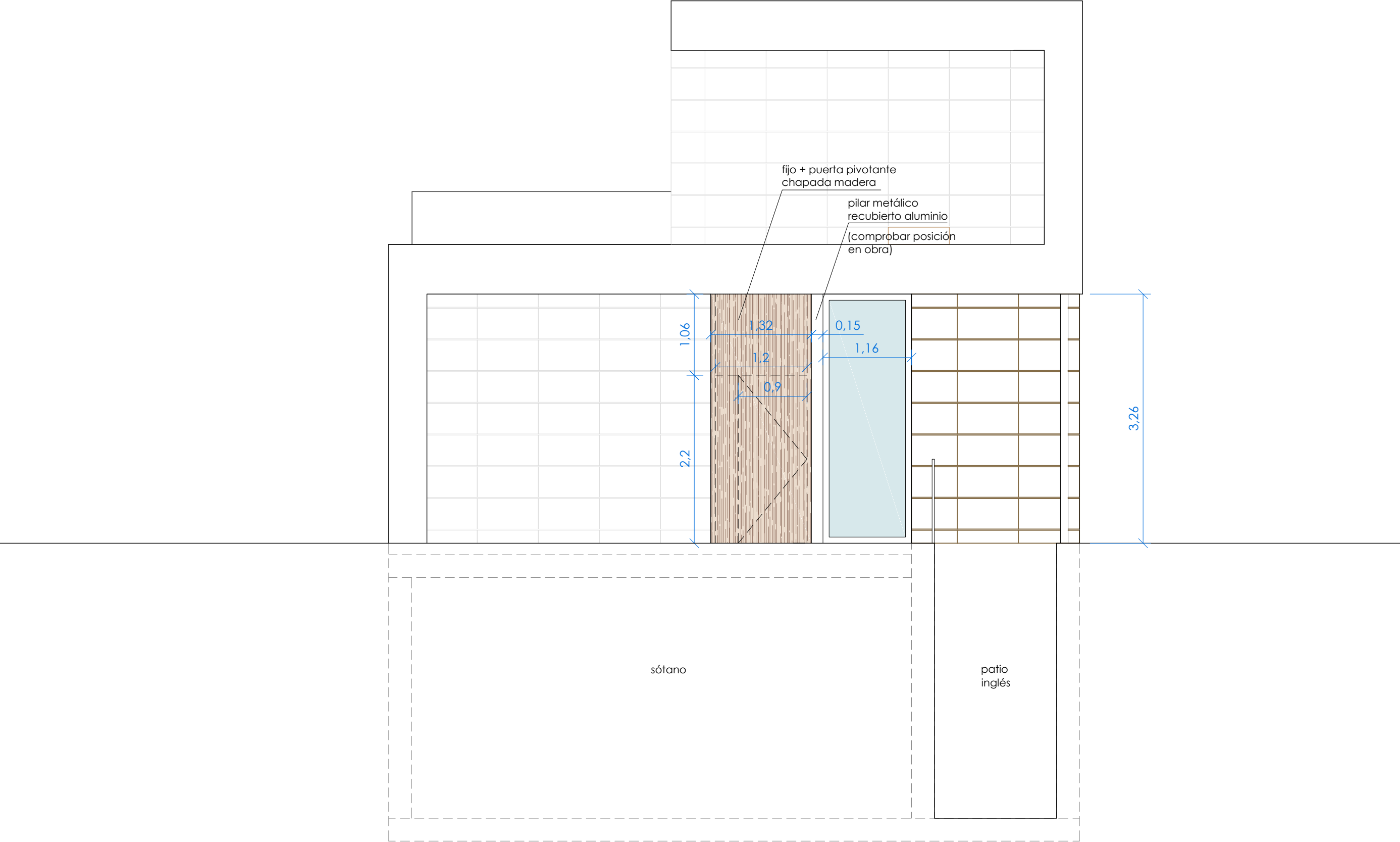
PUERTA ENTRADA VIVIENDA, E:1/50
